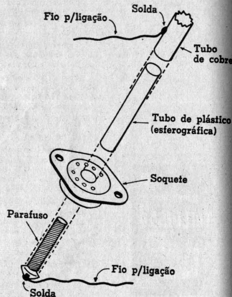
FIG. 2 — Pelo desenho podemos ver a seqüência de encaixes realizados durante a construção do capacitor.
